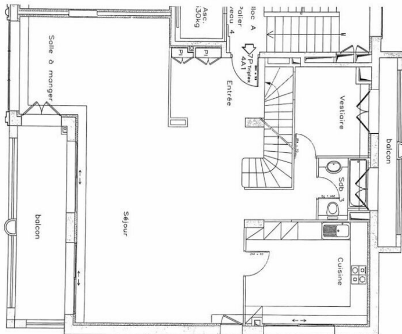
Plan modificatif - Appartements 3A1 + 4A1 - Niveau R+4
